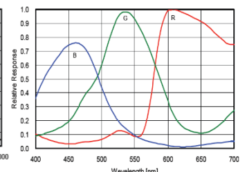
MV-CA030-10GC 量子效率
