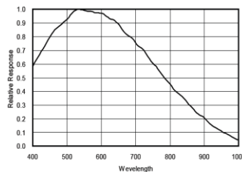
MV-CA030-10GM 量子效率
