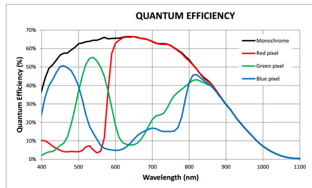
MV-CA013-70GM 量子效率
