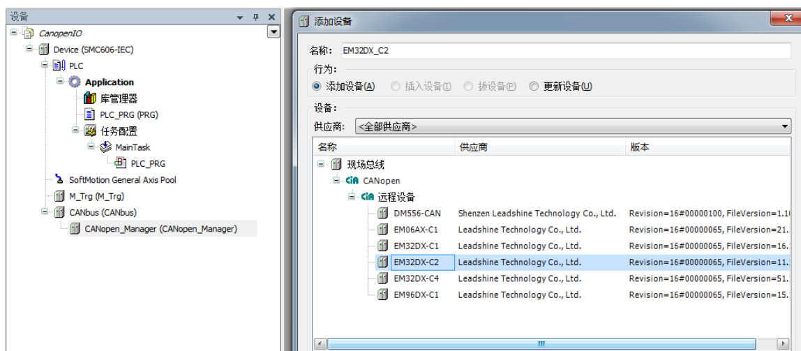
图 4.6 添加EM32DX-A2 模块
