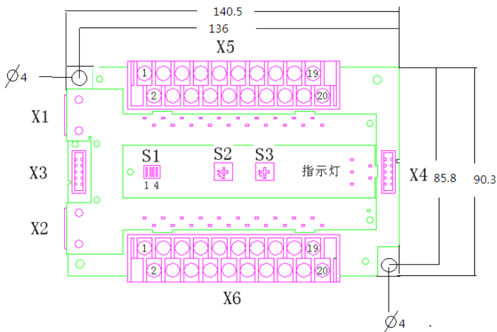
图 3.1 EM32DX-A2 IO扩展模块模块结构尺寸图
