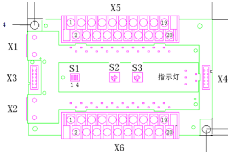
图 2.2 EM32DX-A2 IO 模块硬件接口图
