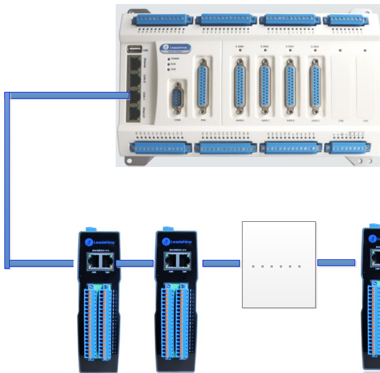
图 5.15 SMC604 和扩展模块连接图
