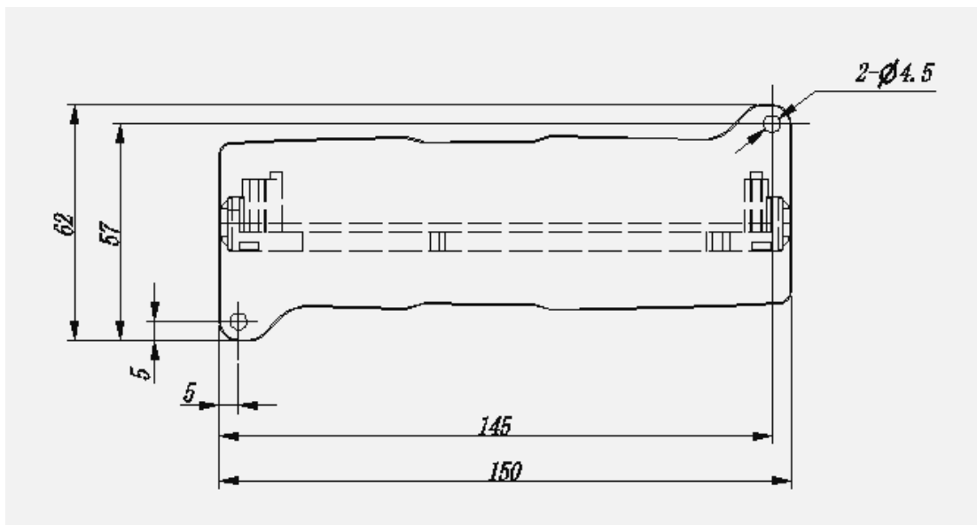
图 1.4 安装底板尺寸图
