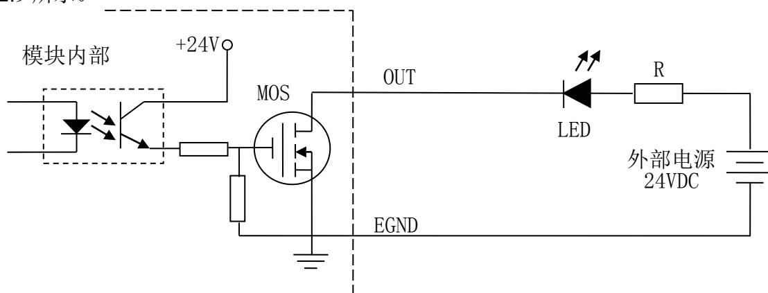
图 2.9 通用输出接线图
