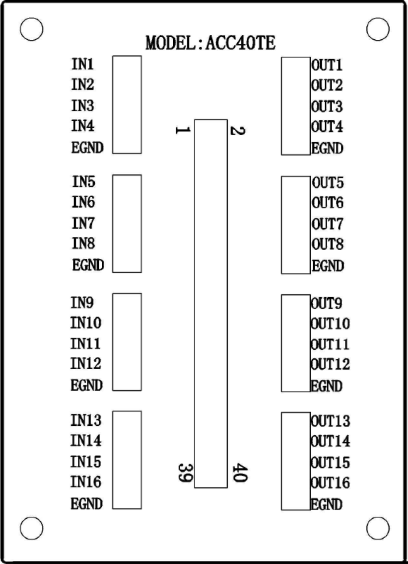
图 2.4 ACC40TE 接线端子引脚分布图
