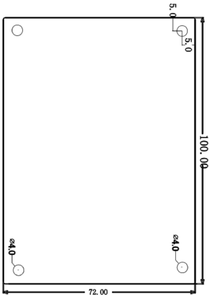
图 2.5 ACC40TE 安装尺寸图
