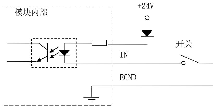
图 2.8 通用输入接线图
