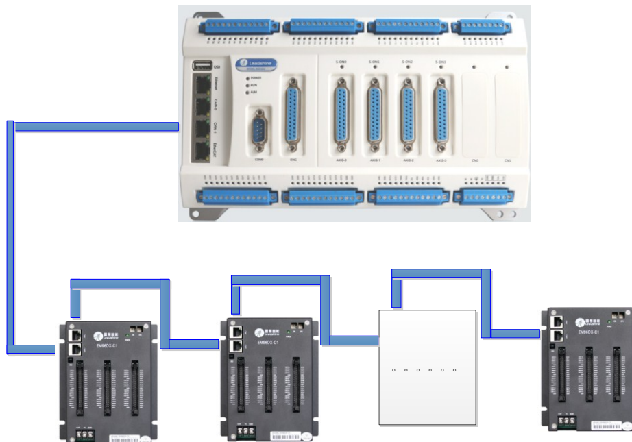
图 5.15 SMC604 和扩展模块连接图
