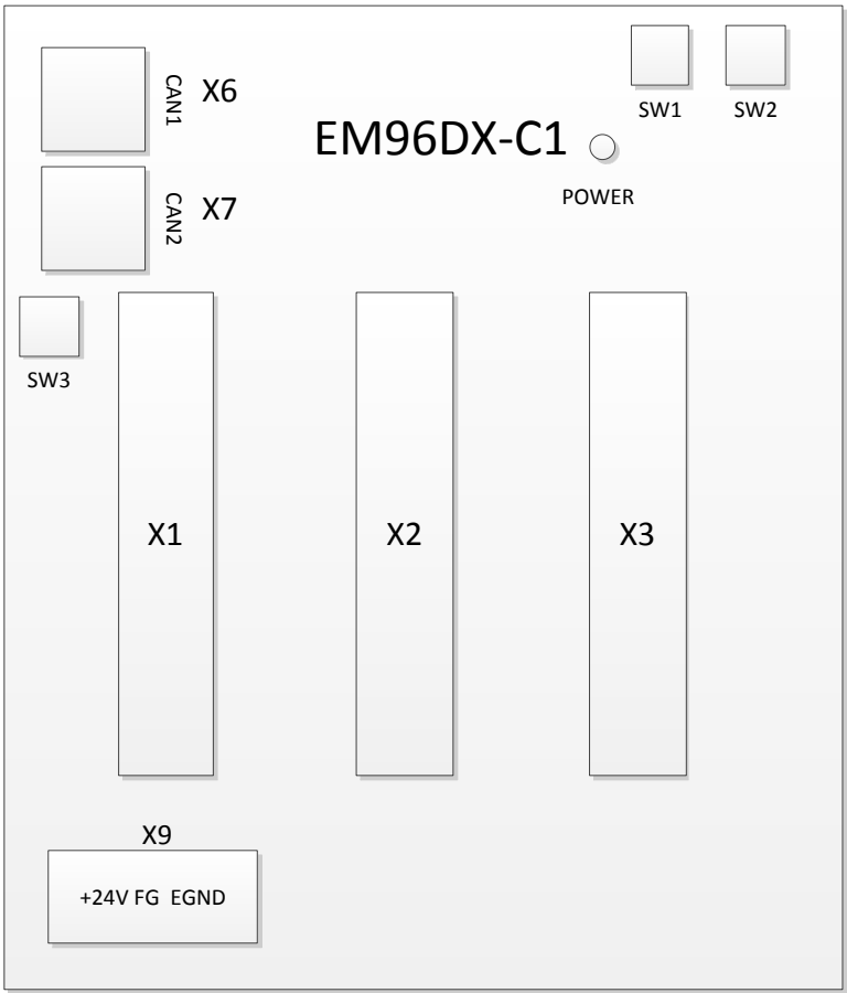
图 2.2 EM96DX-C1 IO 扩展模块硬件接口分布图
