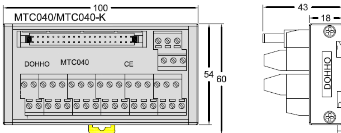
图 2.7 MTC040 端子台安装尺寸图
