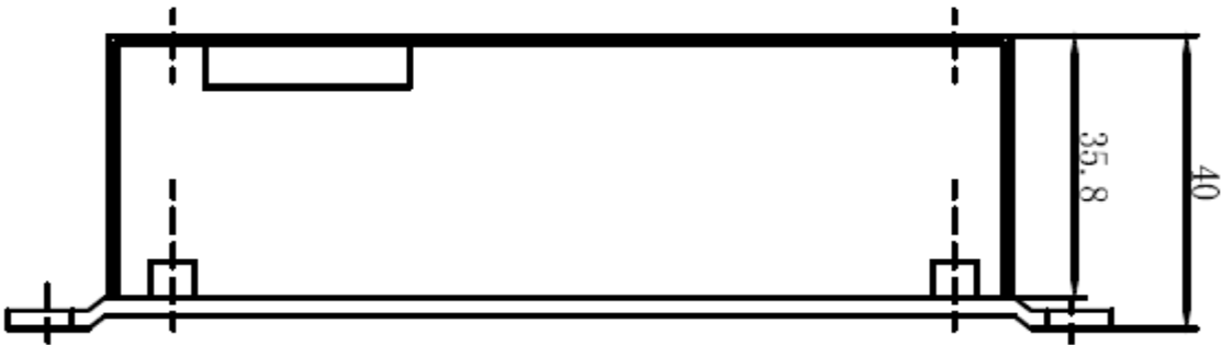
图 1.2 模块侧视图
