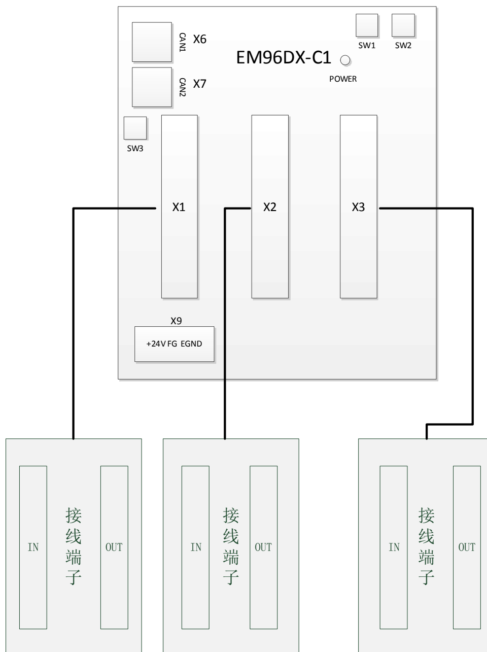
图 2.3 EM96DX-C1 模块和接线端子连接示意图
