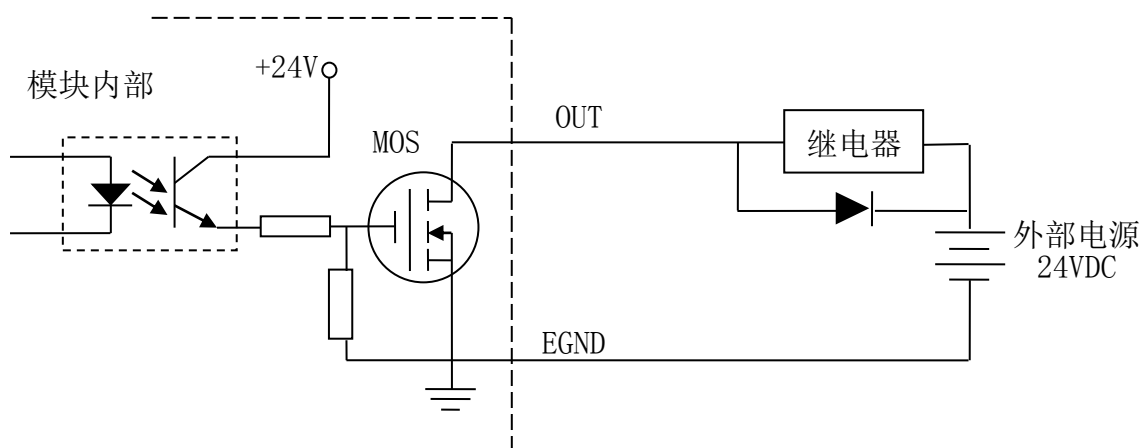
图 2.11 通用输出接线图
