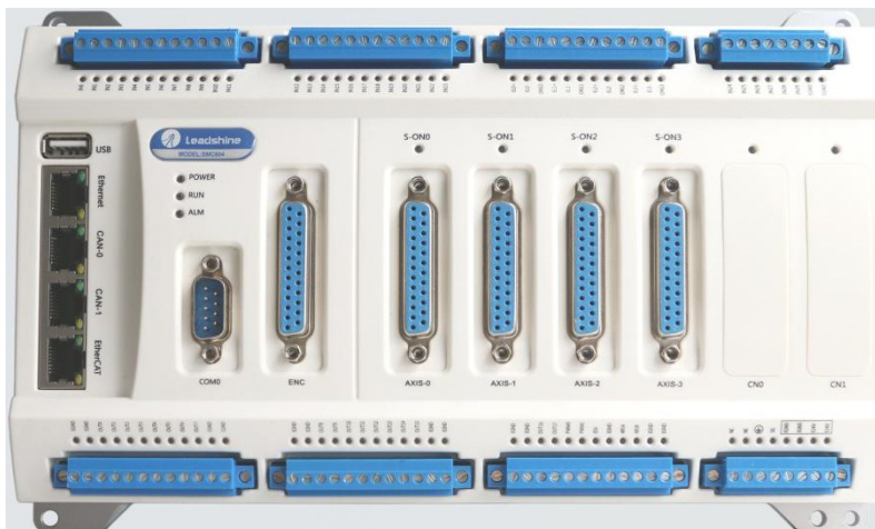
图 5.14 SMC604 外形
