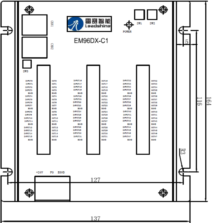
图 1.1 安装底板俯视图
