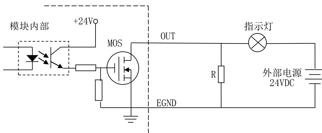
图 2.10 通用输出接线图
