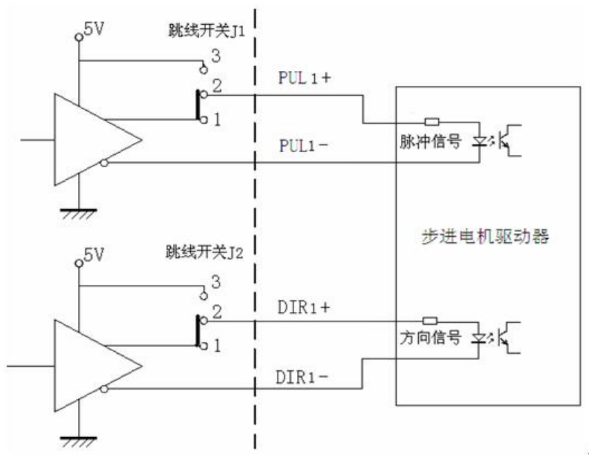
图 5-1 差分方式接线图
