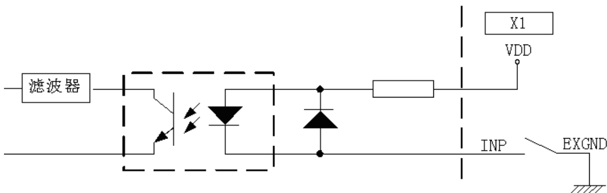
图 5-10 INP 信号输入原理图
