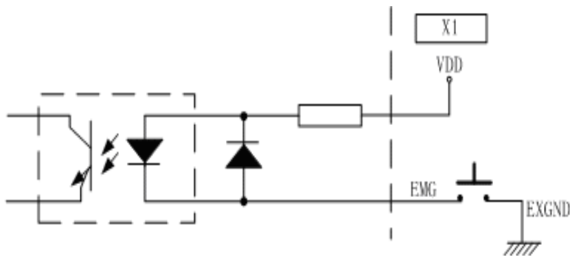
图 5-19 紧急停止输入信号原理图
