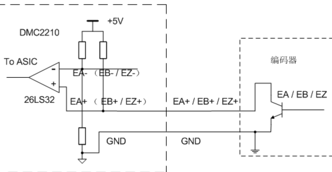
图 5-8 编码器 EA、EB、EZ 信号单端模式原理图
