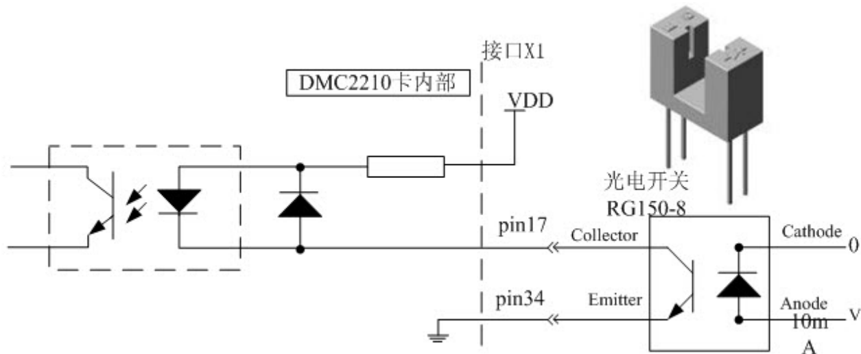
图 6-5 DMC2210 卡与光电开关的接线示例
