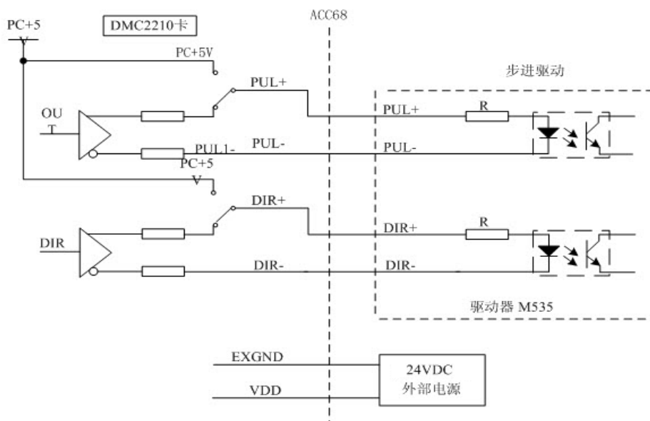
图 6-2 DMC2210 卡与差分步进驱动器的接线
