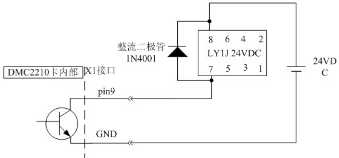
图 6-6 DMC2210 卡与中间继电器的接线示例
