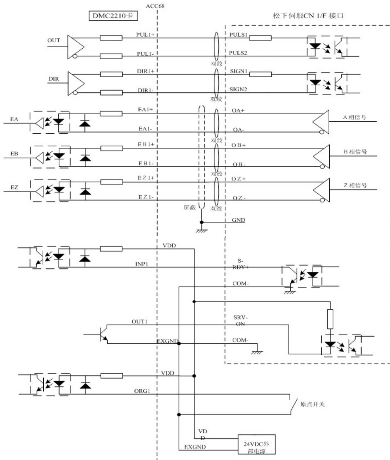
图 6-3 DMC2210 卡与伺服驱动器的接线示例
