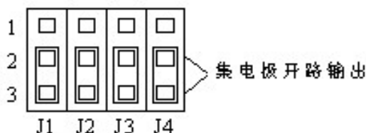
图 3-3 集电极开路输出的跳线设置
