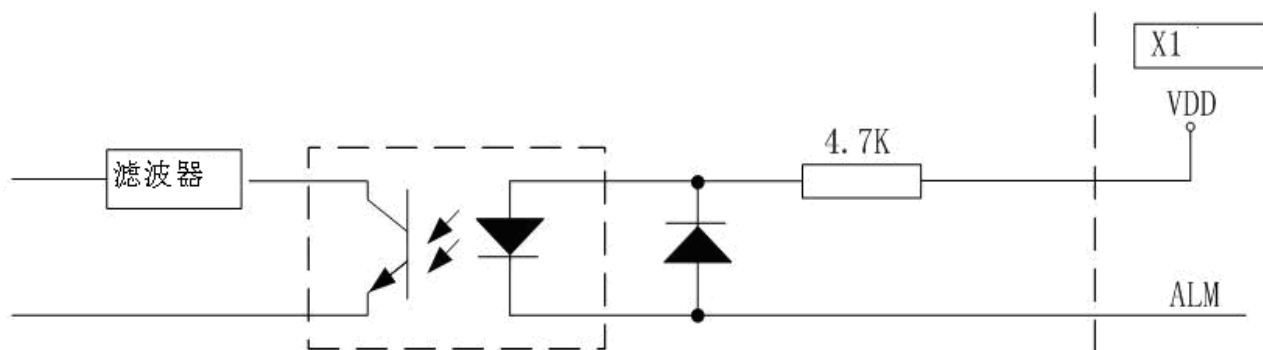
图 5-9 ALM 信号输入原理图
