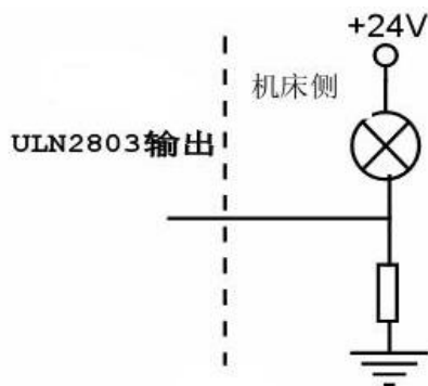
图 5-14 输出口接灯丝型指示灯
