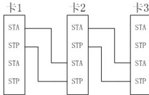
图 4-1 多卡同时启停的连接方式
