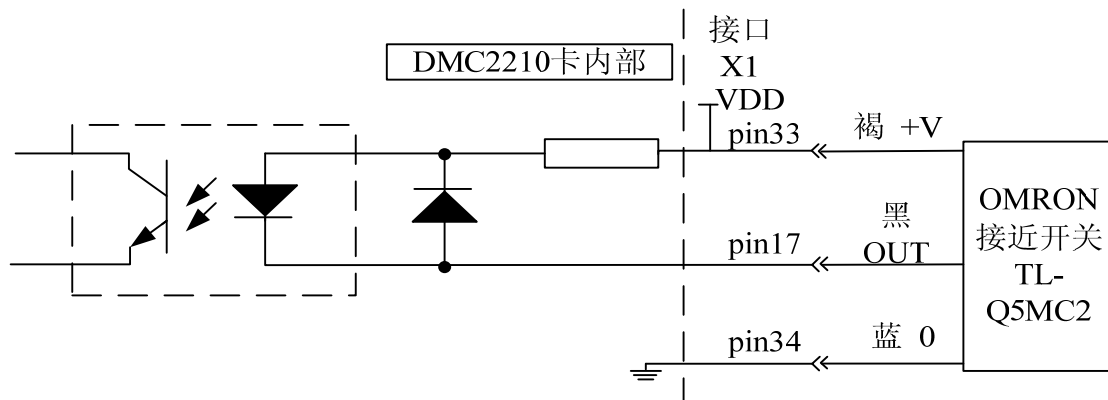
图 6-4 DMC2210 卡与接近开关的接线示例
