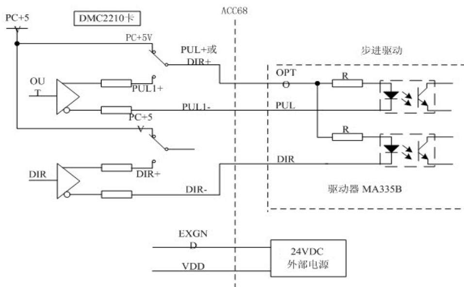
图 6-1 DMC2210 卡与单端步进驱动器的接线
