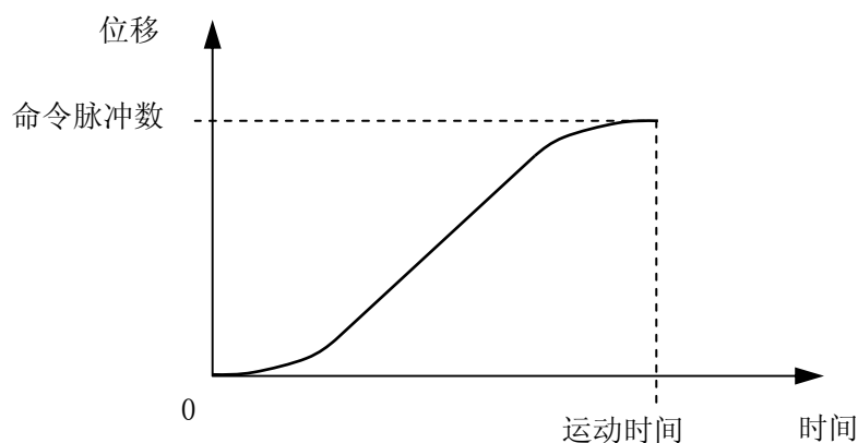
图 2-3 定长运动位移曲线
