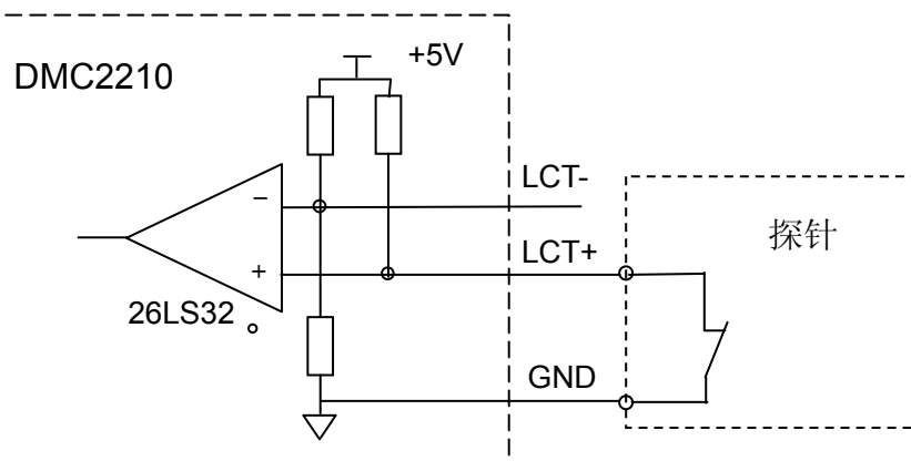
图 5-20 位置锁存输入信号原理图
