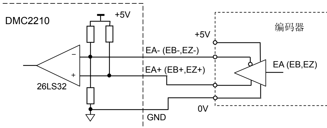
图 5-7 编码器 EA、EB、EZ 信号差分模式原理图
