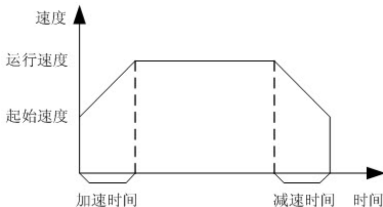
图 2-5 梯形速度曲线
