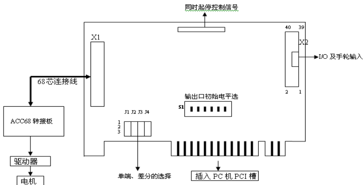
图 3-1 板卡插座和跳线开关布局
