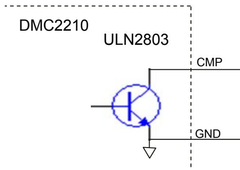
图 5-22 位置比较输出信号接口原理图
