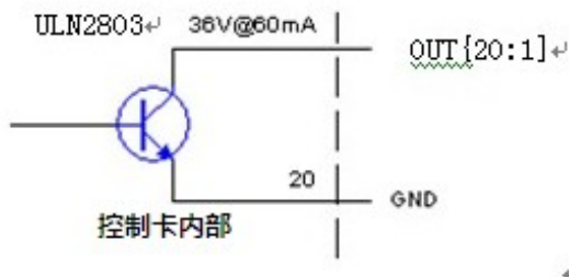
图 5-12 通用数字输出信号输出原理图
