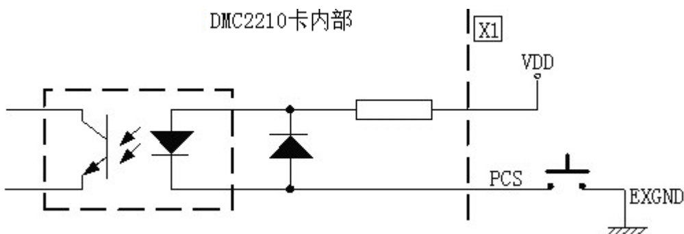
图 5-17 PCS 信号输入原理图
