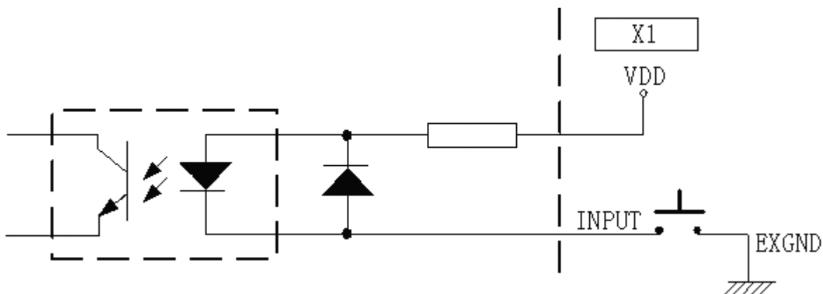
图 5-11 INPUT 信号输入原理图
