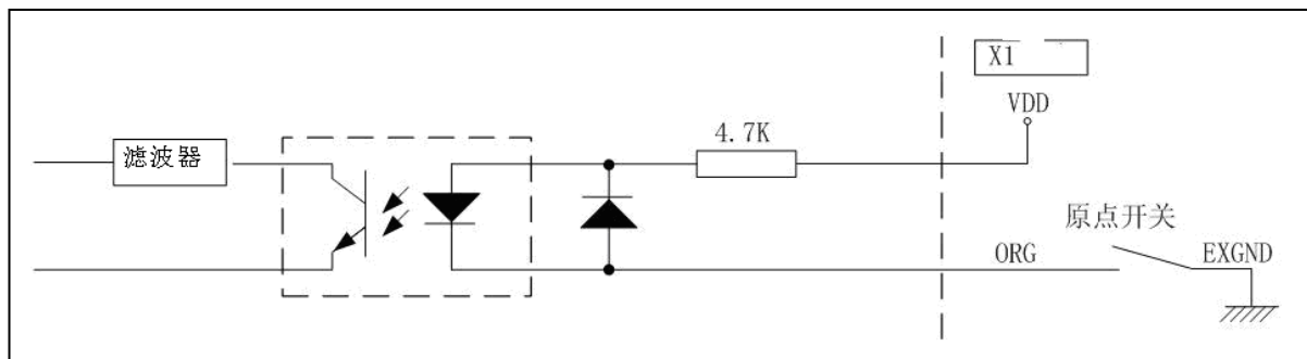
图 5-3 原点信号输入原理图
