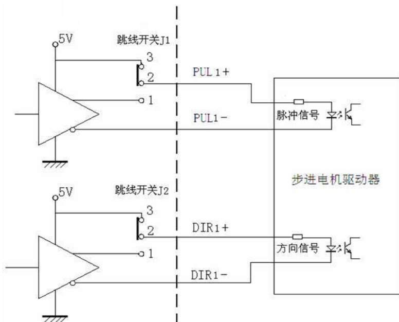
图 5-2 集电极开路方式接线图
