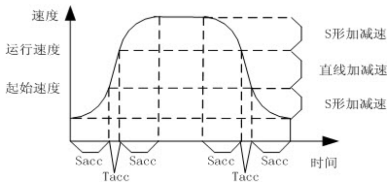
图 2-6 S 形速度曲线
