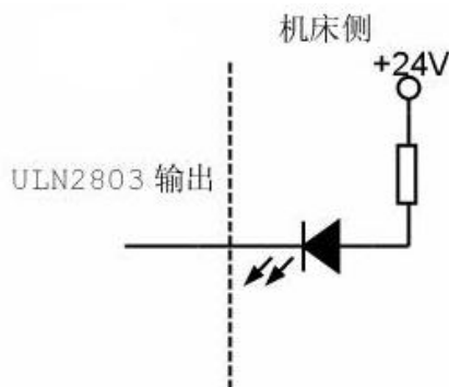
图 5-13 输出口接发光二极管
