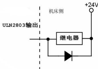
图 5-15 输出口接继电器
