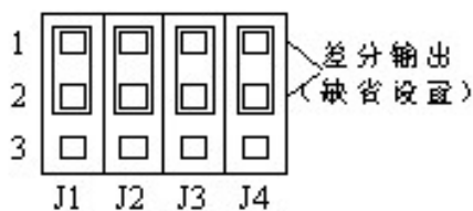
图 3-2 差分输出方式的跳线设置
