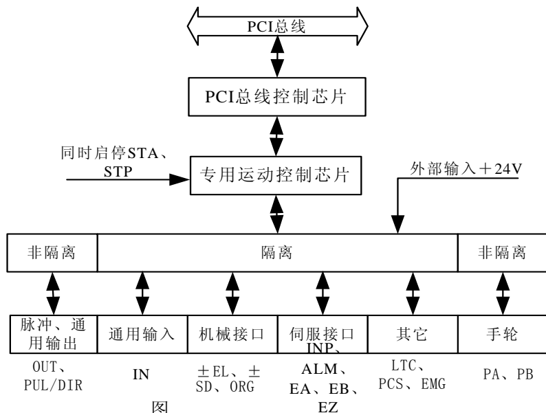
1-1 系统框图
