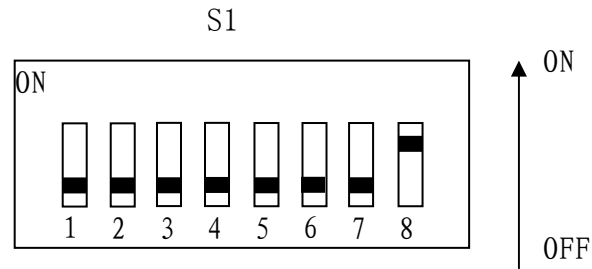
图 3-4 拨码开关 S1 的设置示意图
