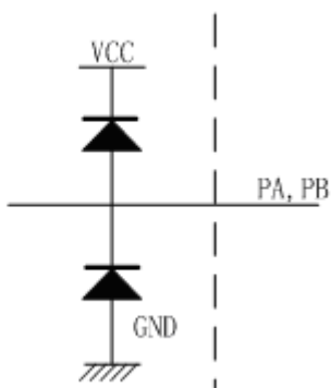
图 5-18 外部脉冲控制信号输入原理图
