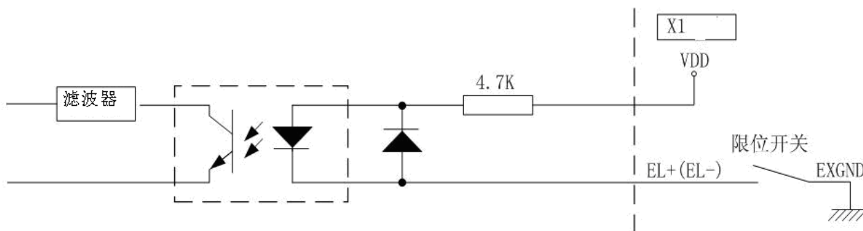
图 5-5 限位信号输入原理图
